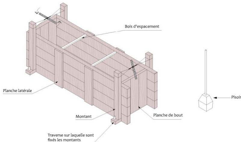
OUTILLAGE DU PISE (Pannaux en Bois)
